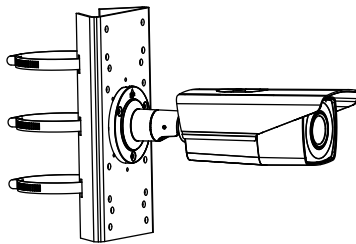
DS-1275ZJ-SUS 垂直ポールマウント
