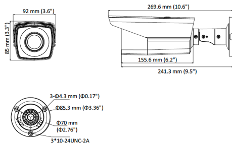
寸法図 (mm)
