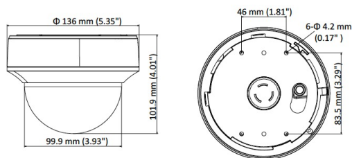
寸法図 (mm)
