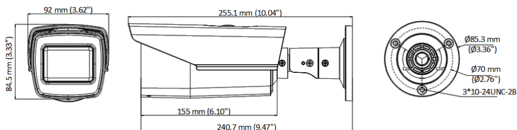
寸法図 (mm)
